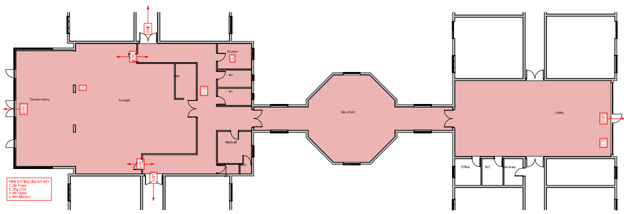
License Plan 1 : 100
